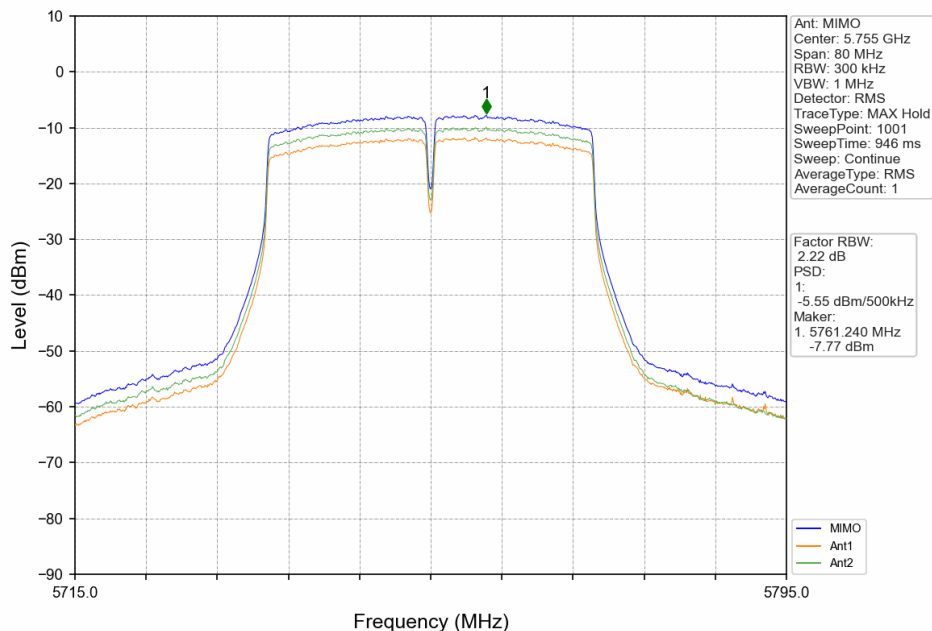
802.11n(HT40)_LCH_5755MHz_MIMO_NTNV
