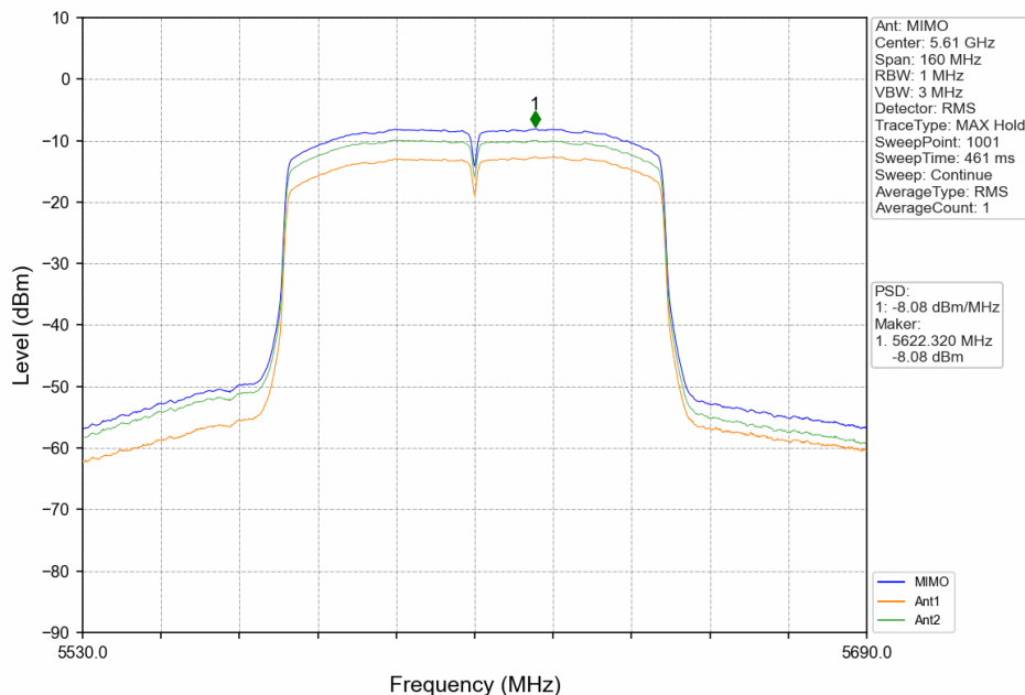
802.11ac(VHT80)_HCH_5610MHz_MIMO_NTNV
