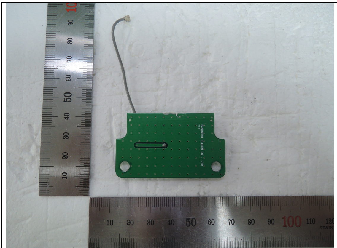
&lt;RFID Antenna&gt;
