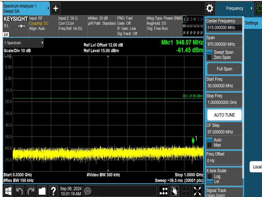
BLE 1M-Ant1-2440-30~1000-PASS
