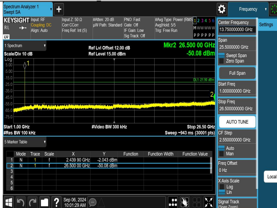
BLE 1M-Ant1-2440-1000~26500-PASS
