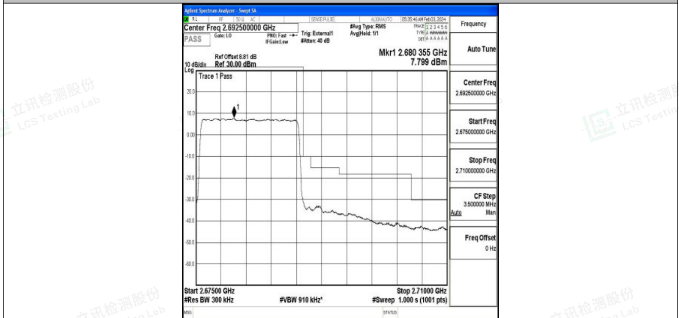
Band41_15MHz_QPSK_41515_75RB#0
