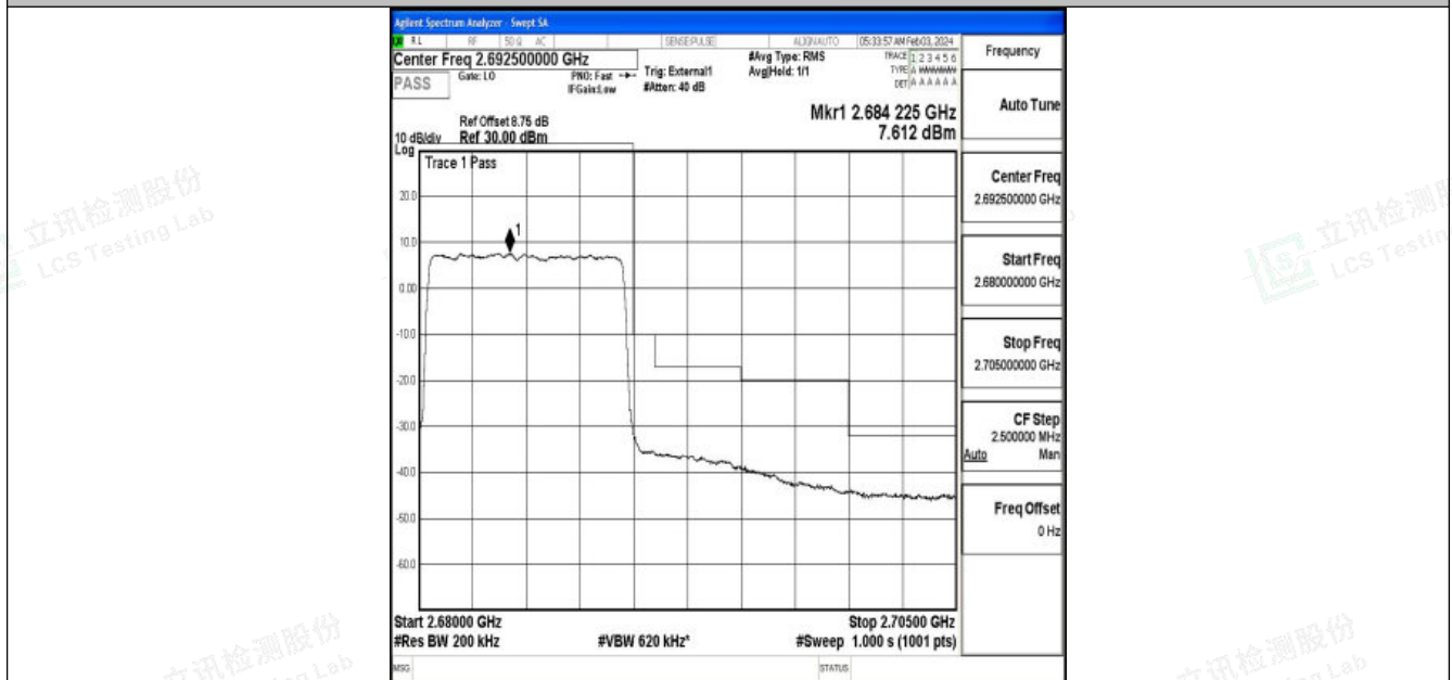
Band41_10MHz_QPSK_41540_50RB#0
