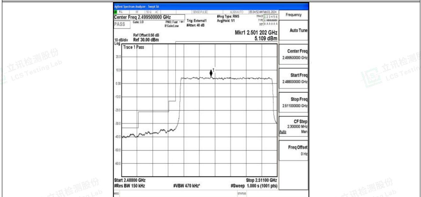
Band41_15MHz_QPSK_39725_75RB#0
