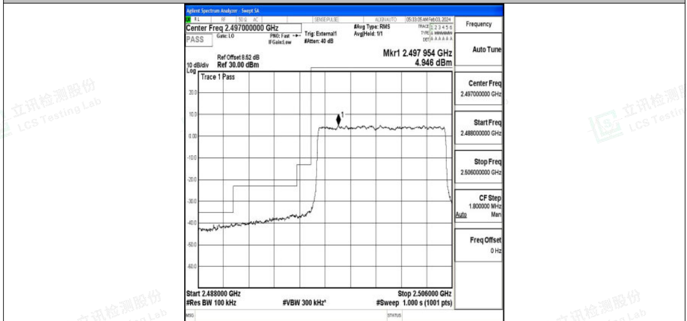
Band41_10MHz_QPSK_39700_50RB#0
