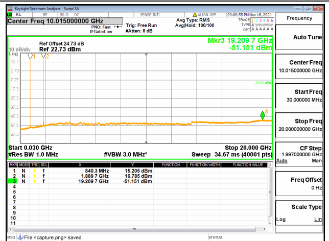
2A-5A / 20+10MHz / QPSK / Mid+High CH / 1@99-1@0
