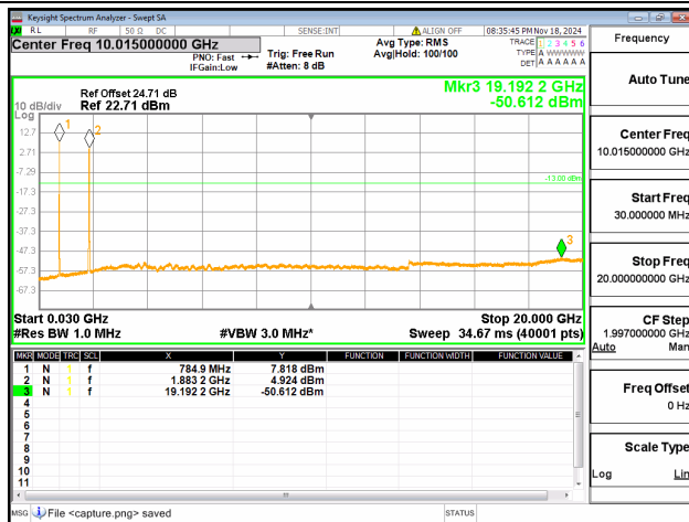
2A-13A / 20+10MHz / QPSK / Mid+Low CH / 100@0-50@0
