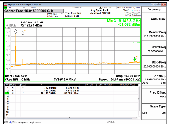
2A-13A / 20+10MHz / QPSK / Mid+Mid CH / 100@0-50@0
