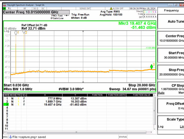
2A-13A / 20+10MHz / QPSK / Mid+Mid CH / 1@99-1@0
