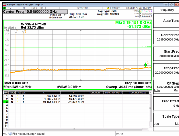
2A-5A / 20+10MHz / QPSK / Mid+Mid CH / 1@99-1@0
