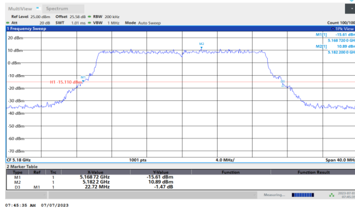
11BE20MIMO_Ant1_5180
