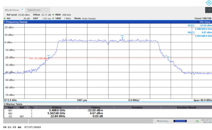
11BE20MIMO_Ant1_5500
