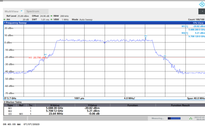
11BE20MIMO_Ant4_5700
