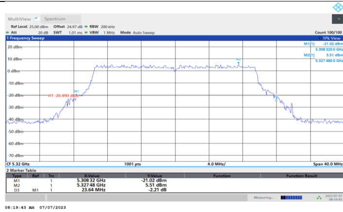
11BE20MIMO_Ant4_5320
