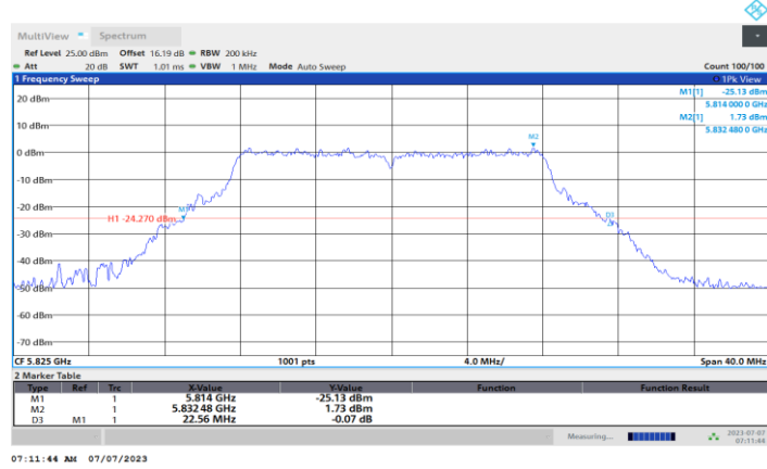
11A-CDD_Ant2_5825
