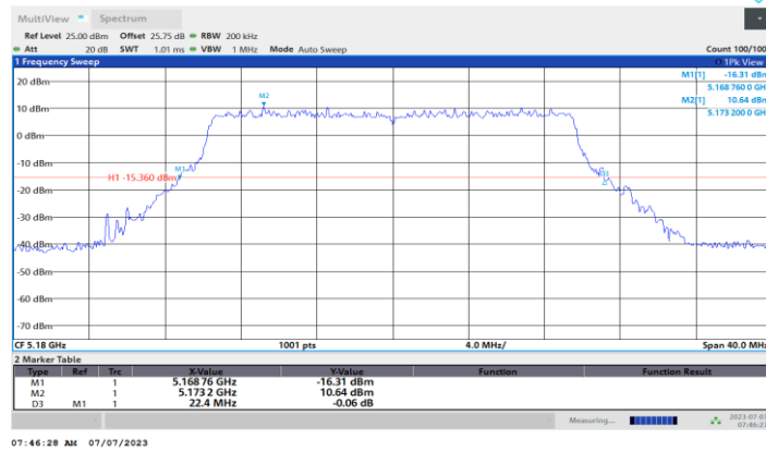
11BE20MIMO_Ant2_5180
