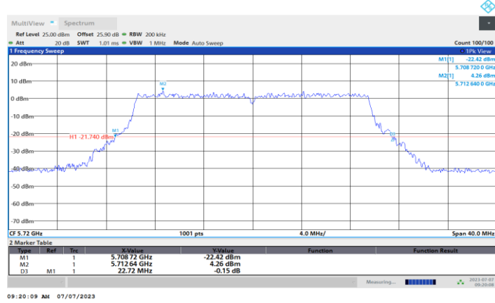
11BE20MIMO_Ant1_5720
