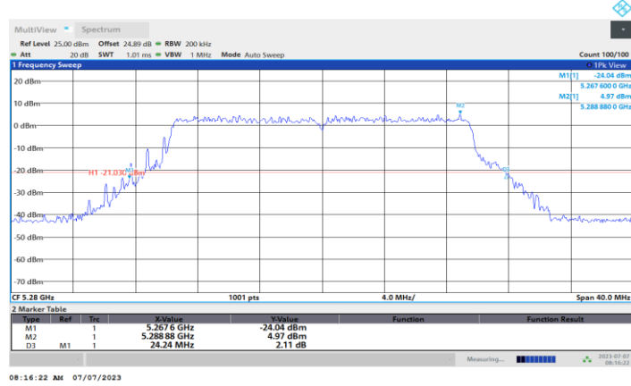
11BE20MIMO_Ant3_5280
