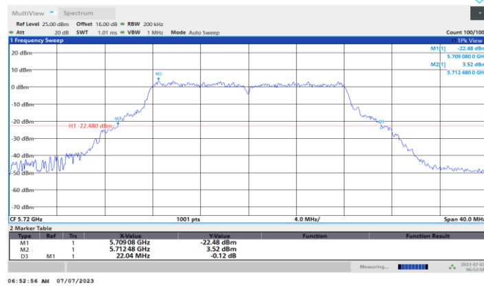
11A-CDD_Ant2_5720
