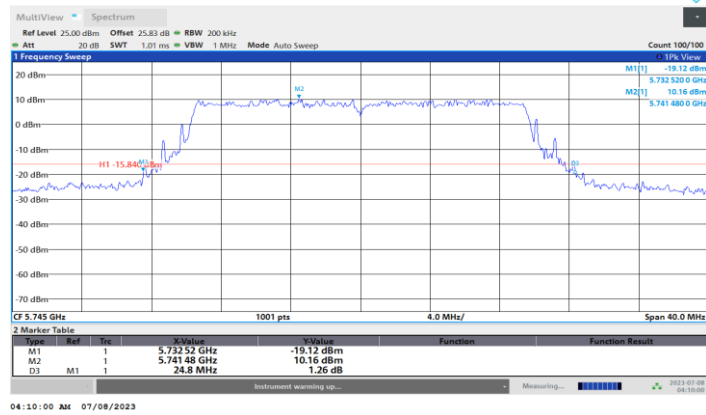
11BE20MIMO_Ant1_5745
