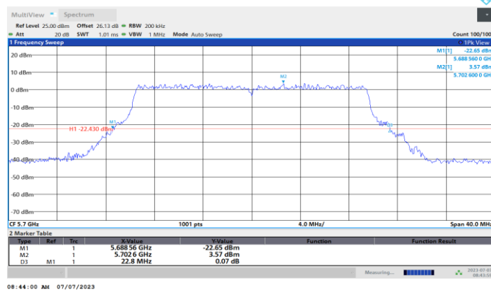
11BE20MIMO_Ant2_5700
