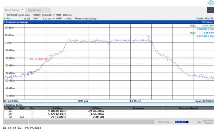
11A-CDD_Ant3_5320
