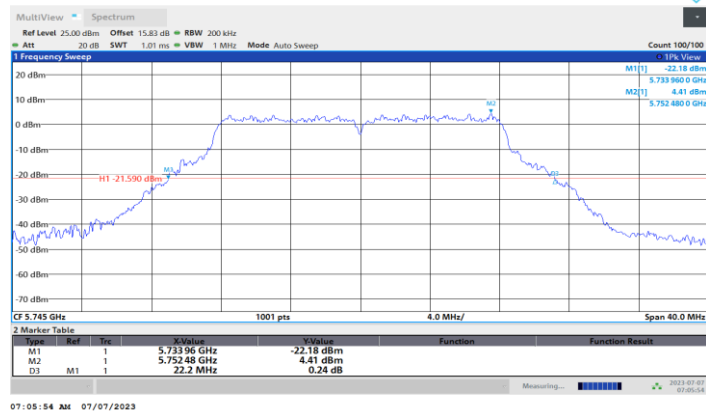
11A-CDD_Ant1_5745
