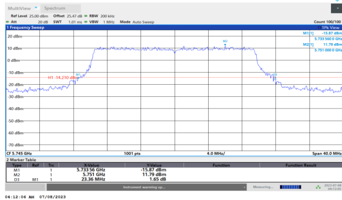
11BE20MIMO_Ant4_5745
