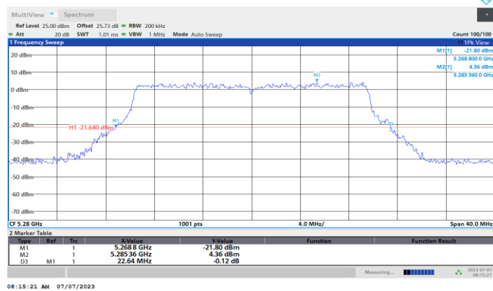
11BE20MIMO_Ant1_5280
