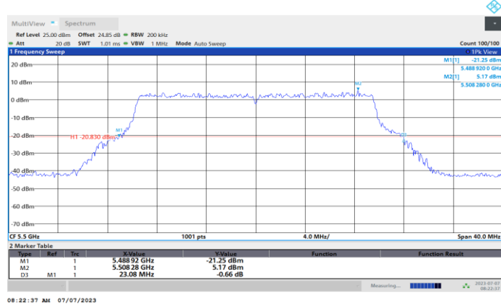
11BE20MIMO_Ant4_5500
