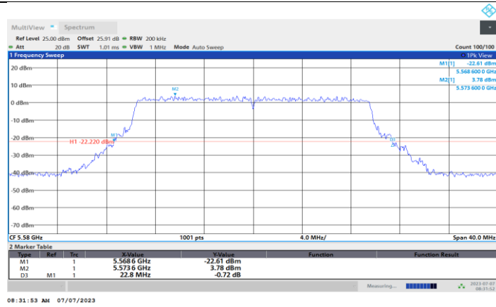
11BE20MIMO_Ant2_5580
