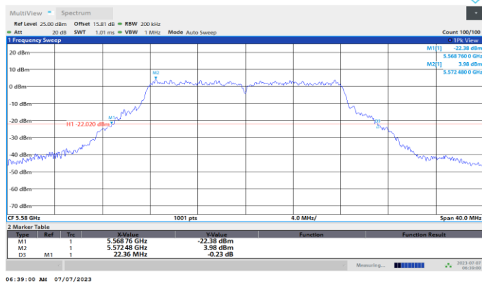
11A-CDD_Ant1_5580
