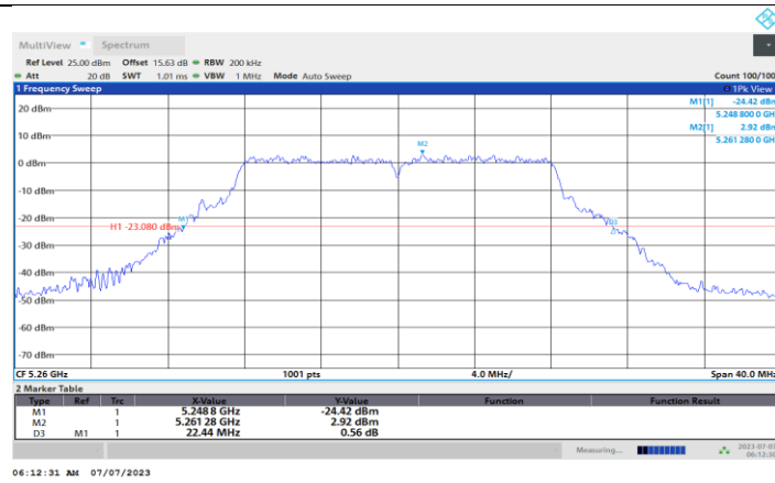
11A-CDD_Ant1_5260
