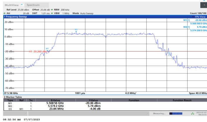
11BE20MIMO_Ant4_5580
