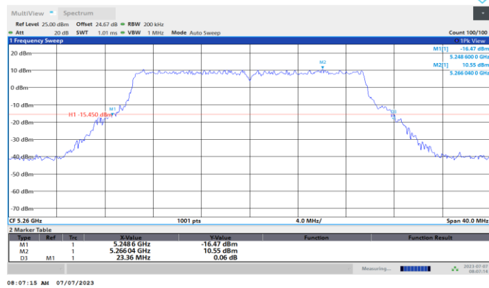
11BE20MIMO_Ant4_5260
