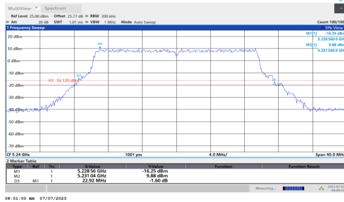
11BE20MIMO_Ant2_5240
