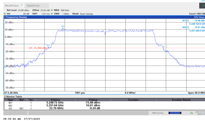
11BE20MIMO_Ant1_5260
