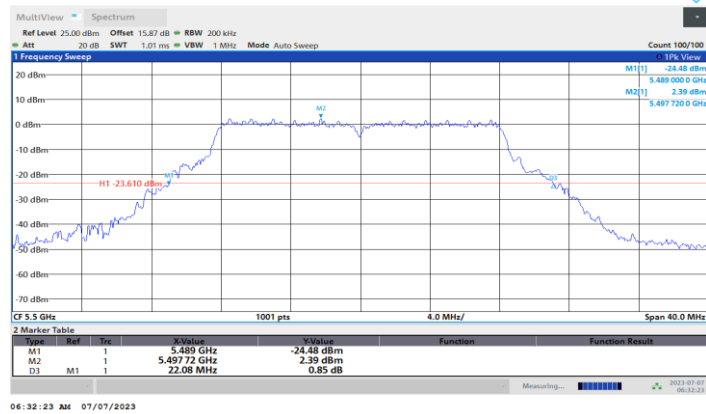
11A-CDD_Ant2_5500
