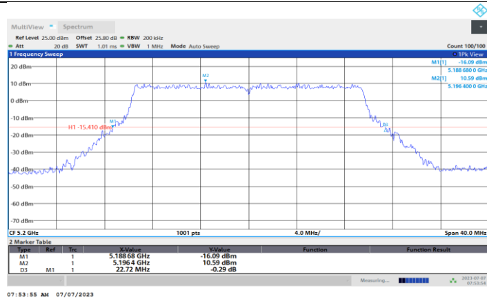
11BE20MIMO_Ant2_5200
