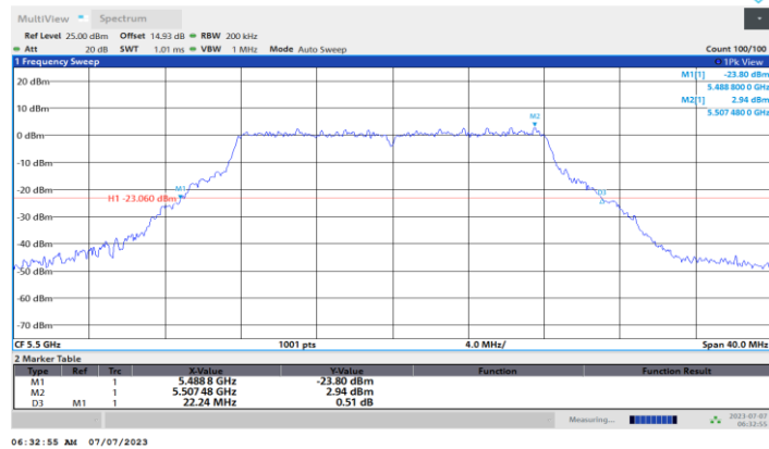
11A-CDD_Ant3_5500
