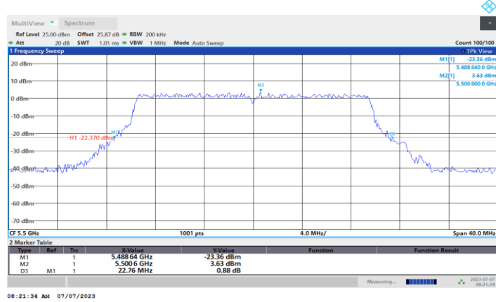
11BE20MIMO_Ant2_5500
