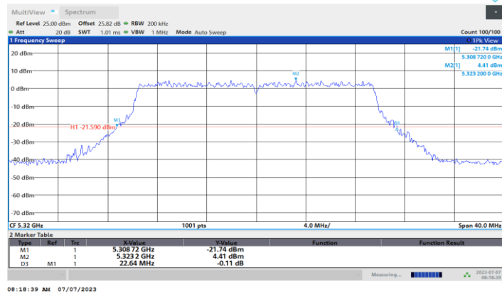
11BE20MIMO_Ant2_5320
