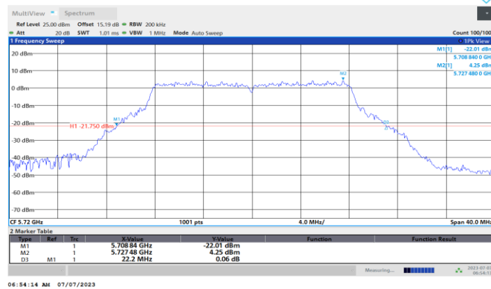
11A-CDD_Ant3_5720
