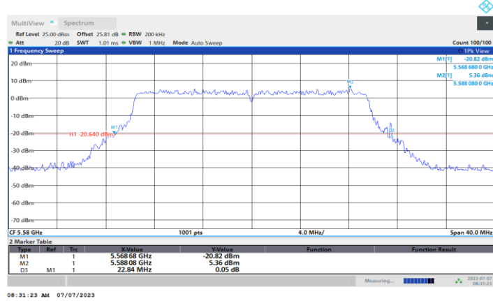
11BE20MIMO_Ant1_5580
