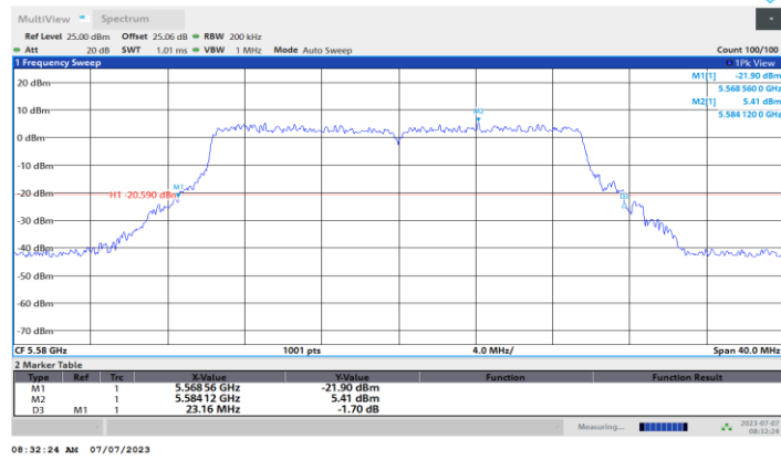
11BE20MIMO_Ant3_5580
