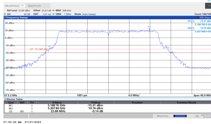
11BE20MIMO_Ant1_5200
