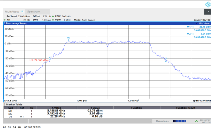
11A-CDD_Ant1_5500
