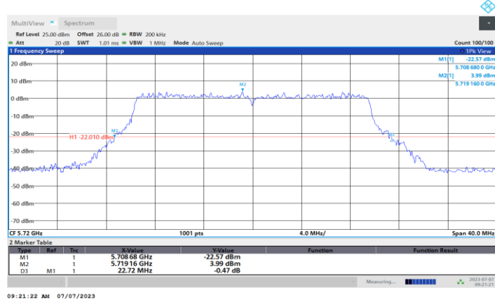
11BE20MIMO_Ant2_5720
