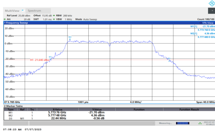
11A-CDD_Ant1_5785
