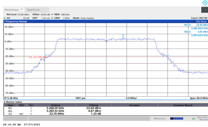
11BE20MIMO_Ant4_5280
