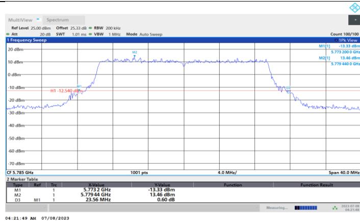
11BE20MIMO_Ant4_5785
