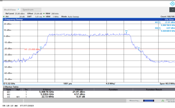
11BE20MIMO_Ant1_5320
