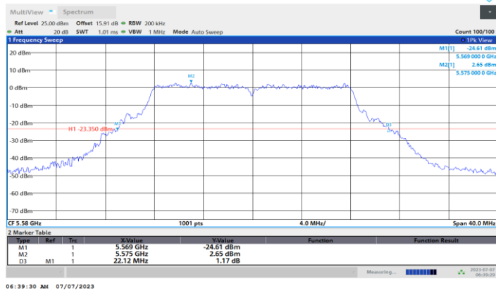
11A-CDD_Ant2_5580
