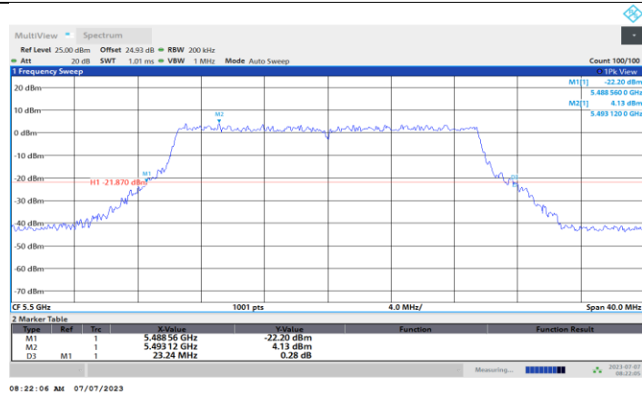
11BE20MIMO_Ant3_5500
