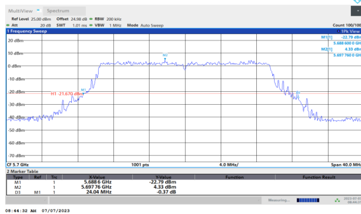
11BE20MIMO_Ant3_5700
