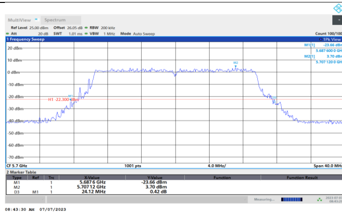
11BE20MIMO_Ant1_5700
