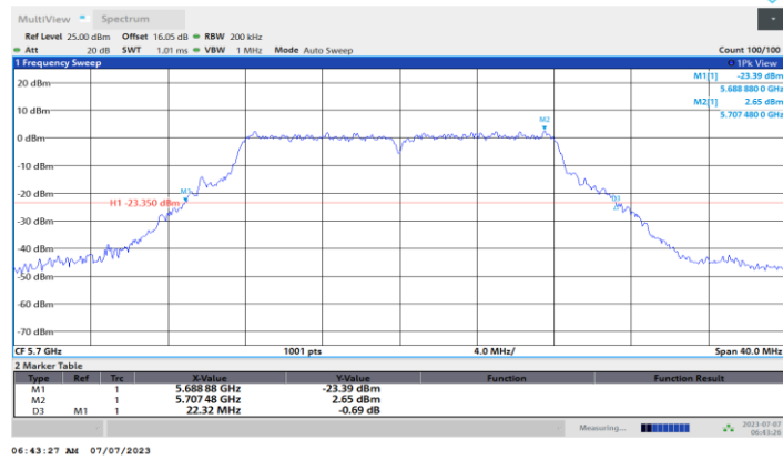
11A-CDD_Ant1_5700
