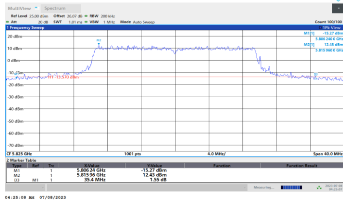
11BE20MIMO_Ant1_5825
