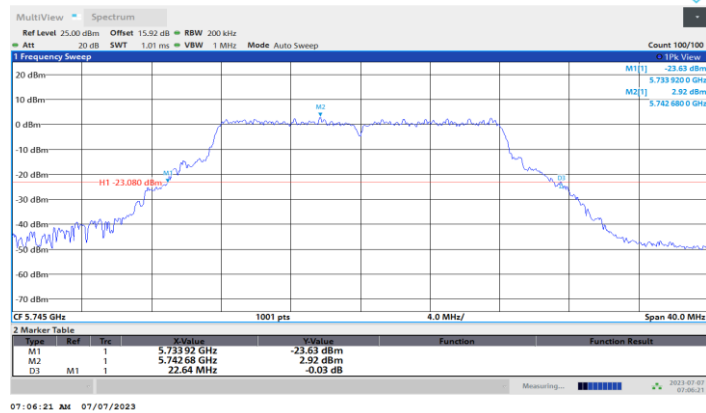
11A-CDD_Ant2_5745
