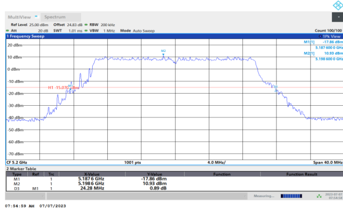
11BE20MIMO_Ant4_5200
