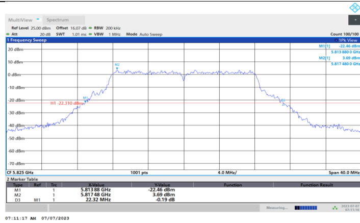
11A-CDD_Ant1_5825
