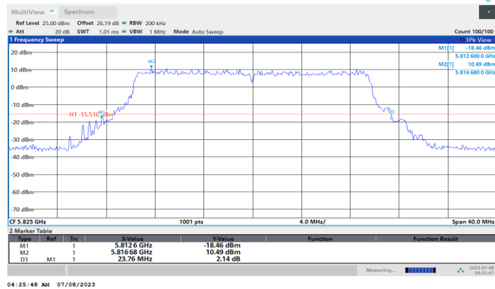
11BE20MIMO_Ant2_5825
