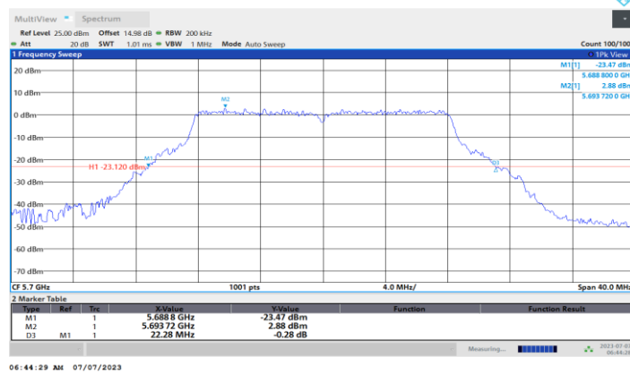
11A-CDD_Ant3_5700
