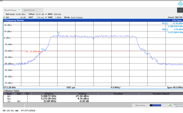
11BE20MIMO_Ant2_5280
