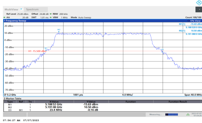
11BE20MIMO_Ant3_5200
