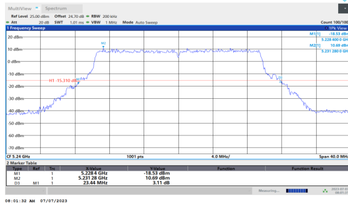
11BE20MIMO_Ant3_5240
