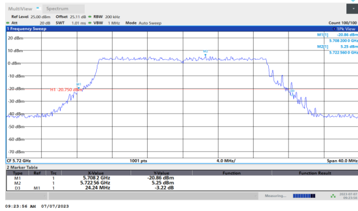
11BE20MIMO_Ant4_5720
