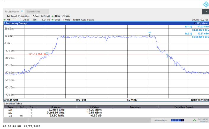
11BE20MIMO_Ant3_5260
