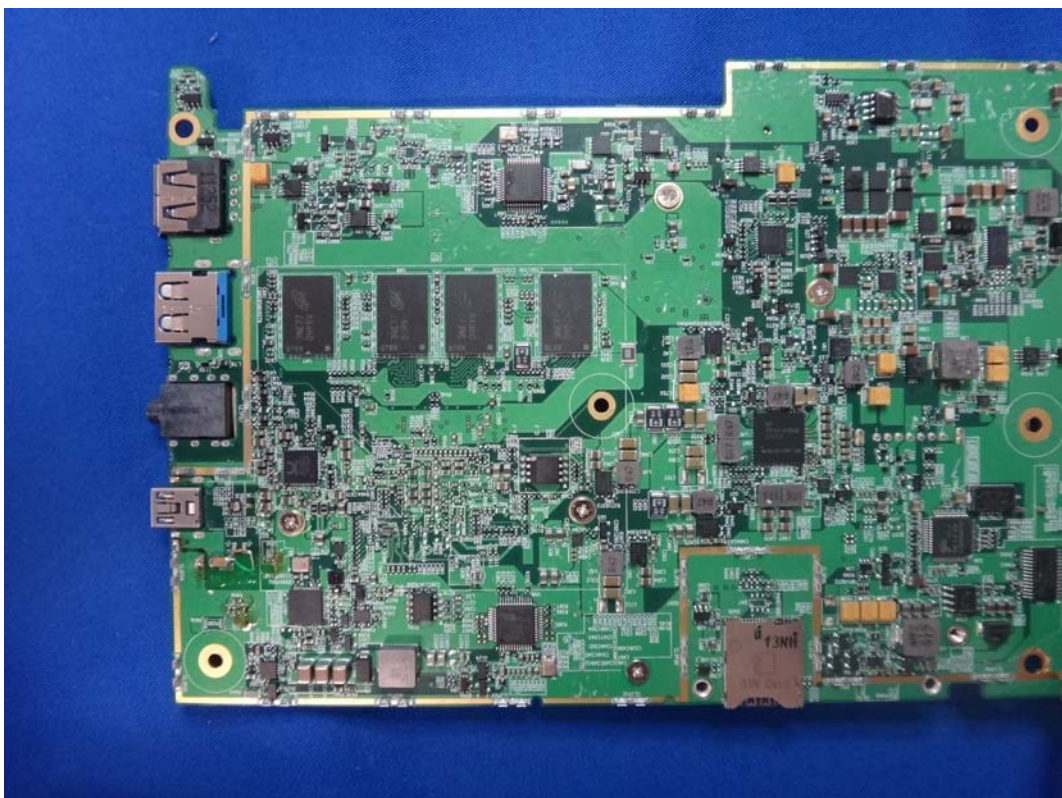
(37) EUT Photo
