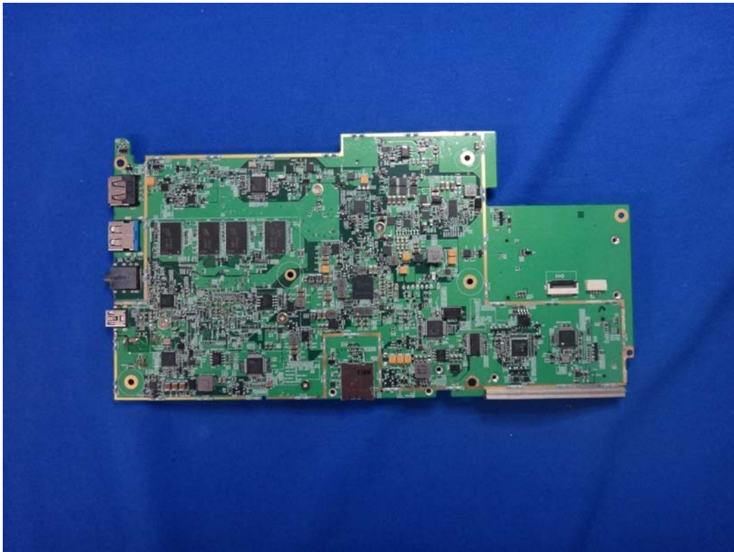
(36) EUT Photo
