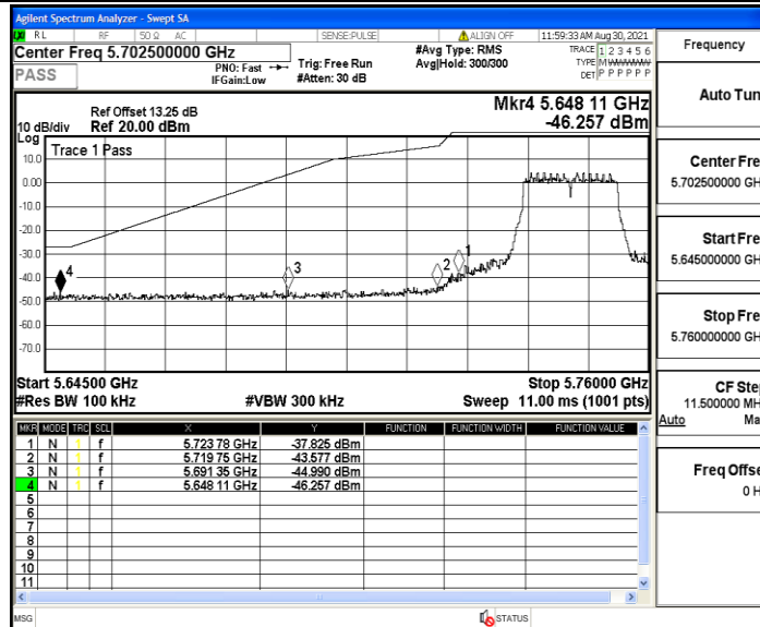
1AC20MIMO_Ant2_Low_5745
