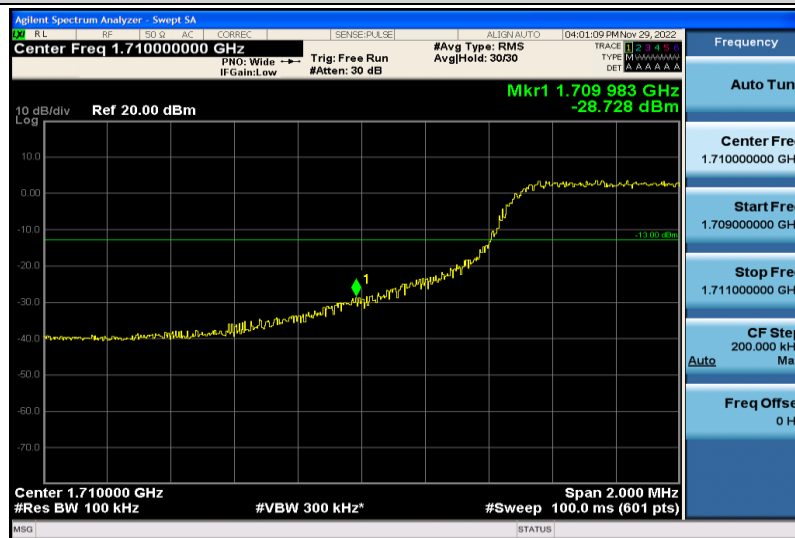
Band66-10MHz-QPSK-132022-50RB#0
