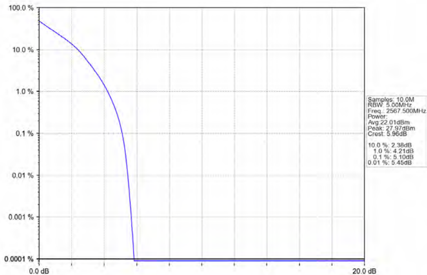
Band7_5MHz_QPSK_HCH_2567.5MHz_RB_25_0_NTNV
