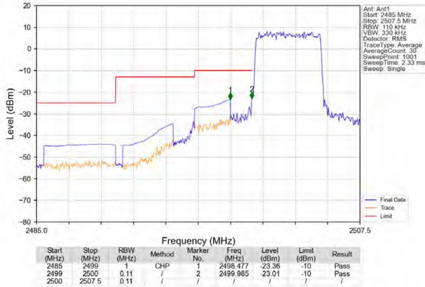
Band7_5MHz_QPSK_LCH_2502.5MHz_RB_25_0_NTNV
