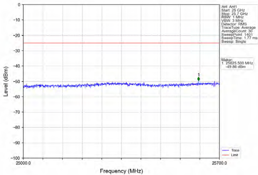
Band7_15MHz_QPSK_HCH_2562.5MHz_RB_1_74_NTNV
