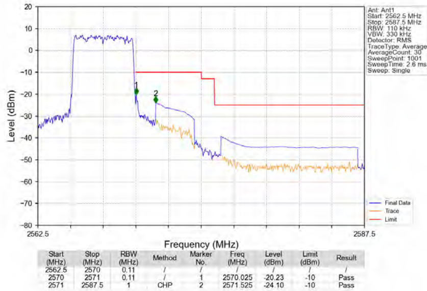
Band7_5MHz_QPSK_HCH_2567.5MHz_RB_25_0_NTNV
