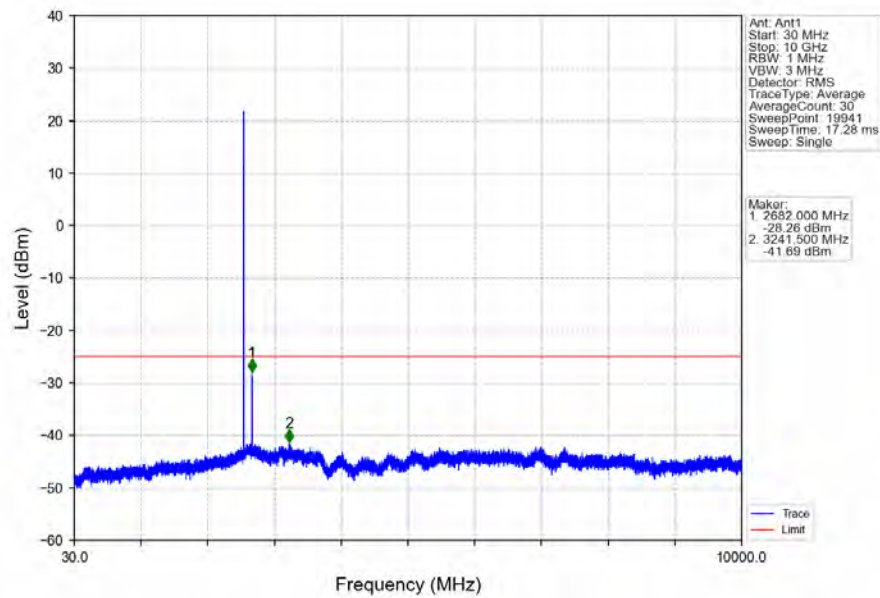
Band7_10MHz_QPSK_HCH_2565MHz_RB_1_0_NTNV
