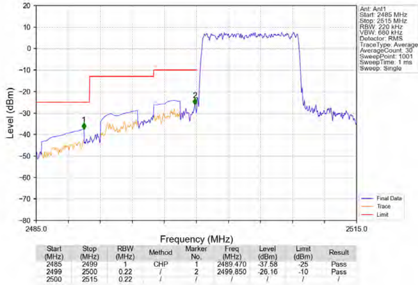
Band7 10MHz QPSK LCH 2505MHz RB 50 0 NTNV
