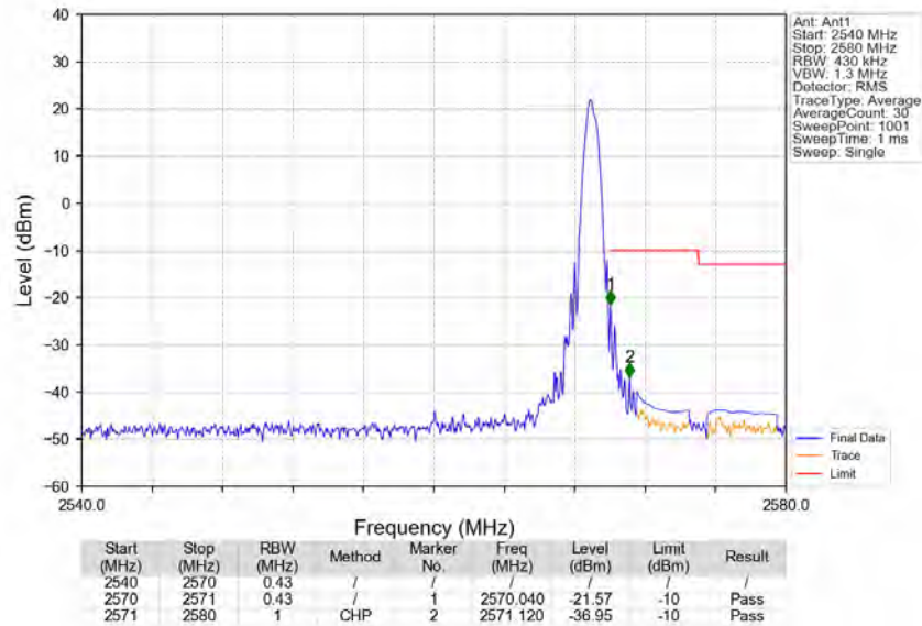
Band7_20MHz_16QAM_HCH_2560MHz_RB_1_99_NTNV
