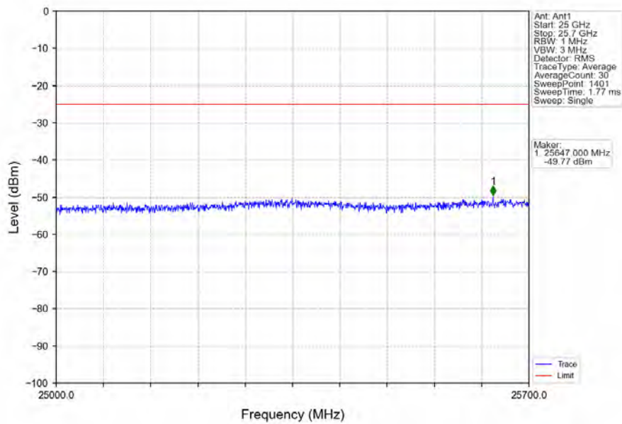
Band7_5MHz_QPSK_HCH_2567.5MHz_RB_1_24_NTNV
