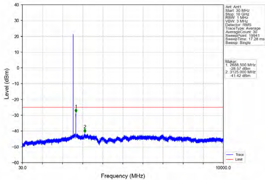
Band7_20MHz_QPSK_HCH_2560MHz_RB_1_0_NTNV
