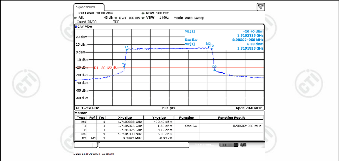
Band4-10MHz-QPSK-20000-50RB#0-8.985
