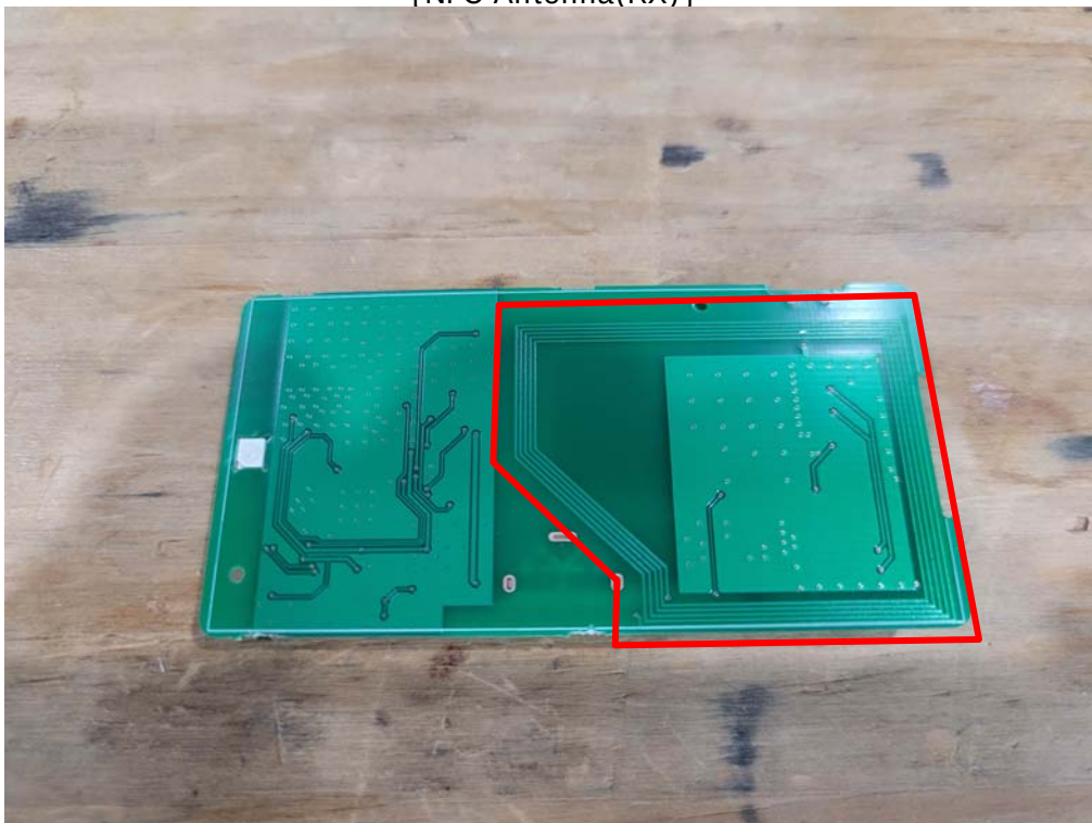
{ NFC Antenna(RX) }
