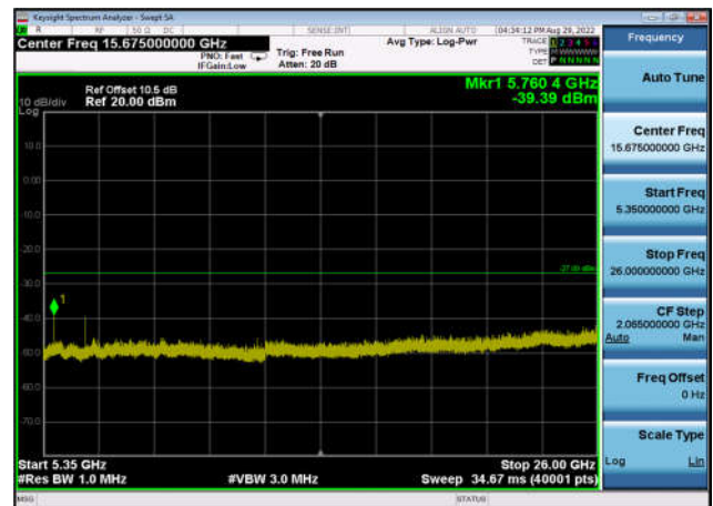
U-NII-1 ,Plot 3,5350MHz~26000MHz-802. 11n(20MHz),5220MHz,Ant1
