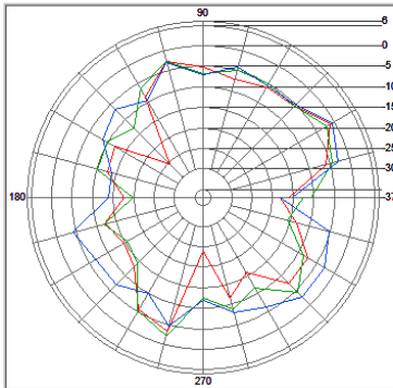
Ant 1, Theta, XZ-Plan
