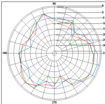
Ant 1, Theta, YZ-Plan
