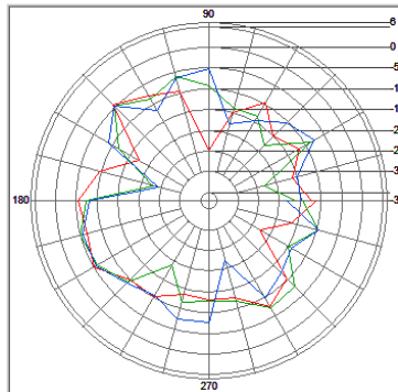
Ant 2, Phi, YZ-Plan
