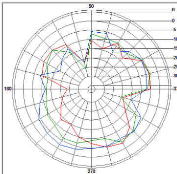
Ant 1, Theta, XY-Plan
