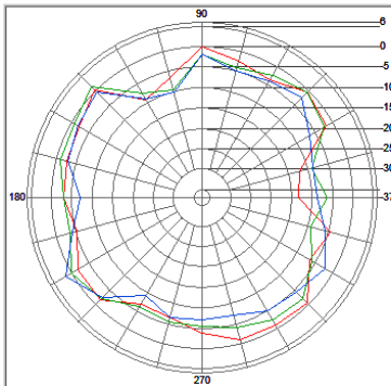
Ant 2, Theta, XY-Plan
