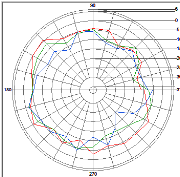
Ant 3, Theta, XZ-Plan
