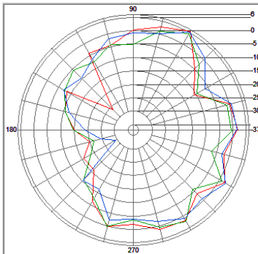
Ant 3, Theta, YZ-Plan
