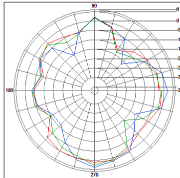
Ant 1, Phi, XZ-Plan
