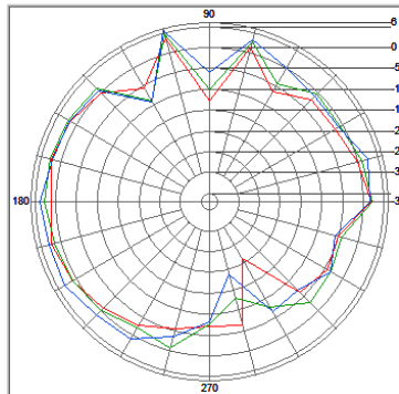
Ant 1, Phi, XY-Plan
