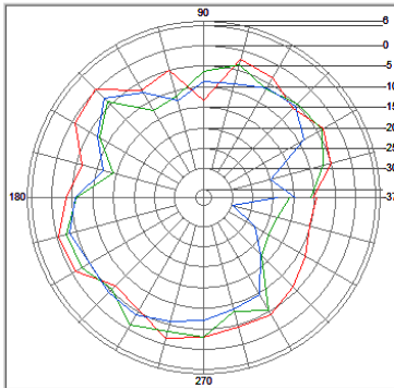
Ant 2, Theta, XZ-Plan
