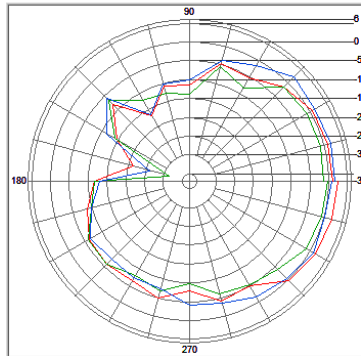
Ant 2, Phi, XZ-Plan
