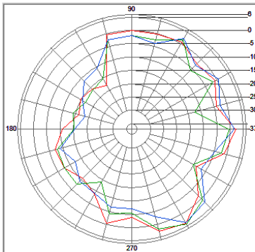
Ant 2, Theta, YZ-Plan
