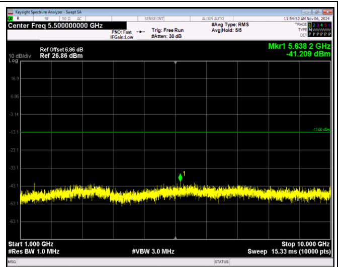
Band12-10MHz-QPSK-23130-1RB#0-Range2:1000~1 0000MHz
