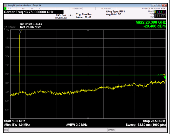
Band7-5MHz-16QAM-21425-1RB#0-Range2:1000~26 500MHz
