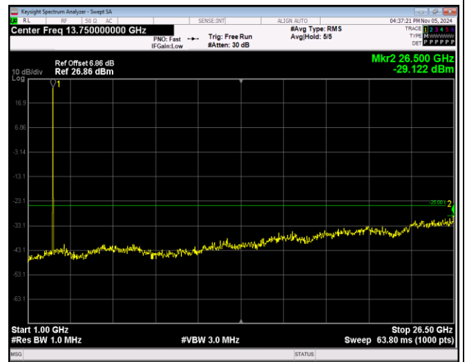
Band7-20MHz-QPSK-21100-1RB#0-Range2:1000~26 500MHz
