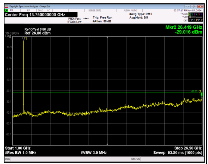
Band7-5MHz-QPSK-20775-1RB#0-Range2:1000~265 00MHz
