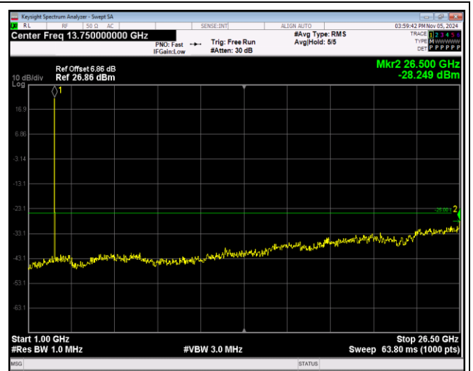
Band7-20MHz-QPSK-20850-1RB#0-Range2:1000~26 500MHz
