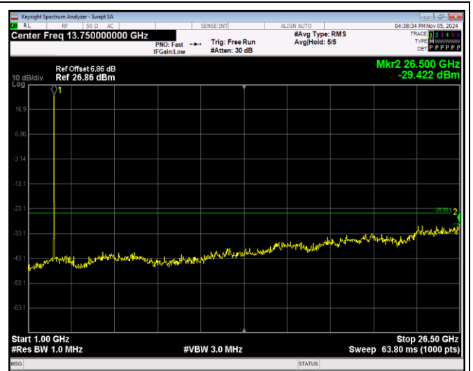
Band7-20MHz-16QAM-21350-1RB#0-Range2:1000~2 6500MHz
