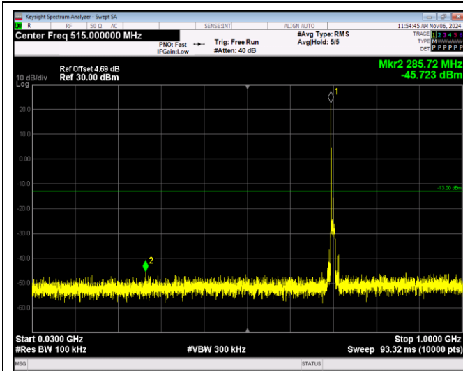
Band12-10MHz-QPSK-23130-1RB#0-Range1:30~100 OMHz
