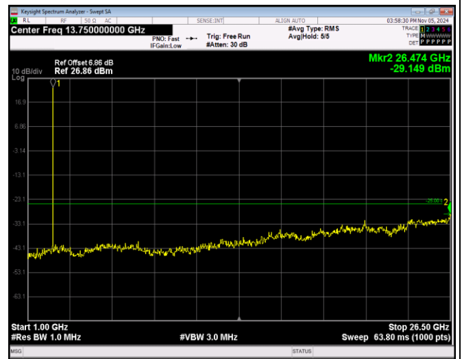
Band7-5MHz-16QAM-21425-1RB#0-Range2:1000~26 500MHz
