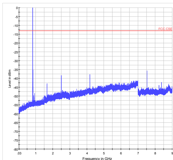
GSM 850 CH-Middle 30MHz~9GHz
