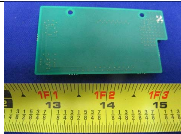
LMA M6e RFID Module Bottom View
