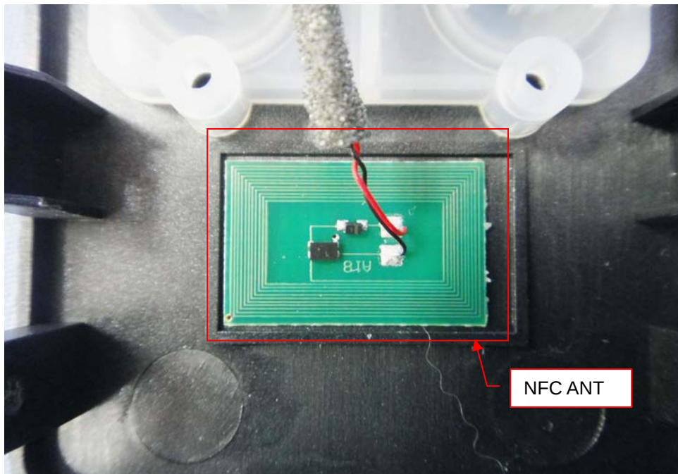
EUT Photo 20 )
