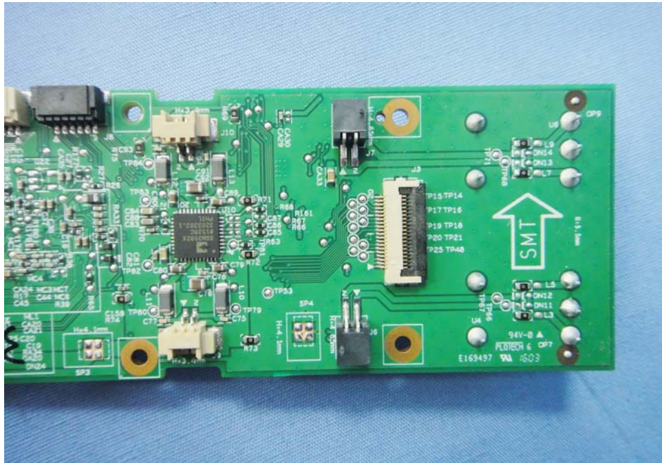
EUT Photo 8 )
