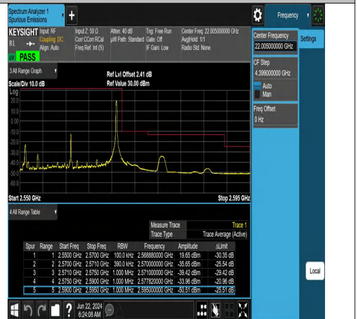
Band7-20MHz-QPSK-21350-1RB#99-PASS
