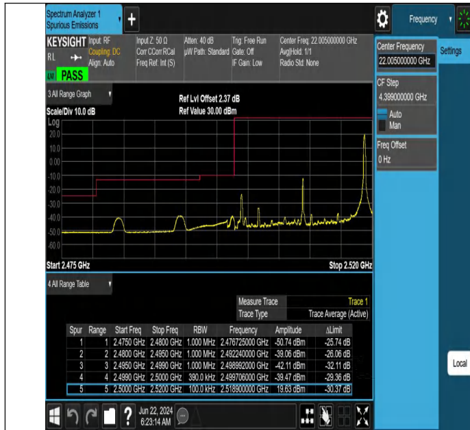
Band7-20MHz-QPSK-20850-1RB#99-PASS
