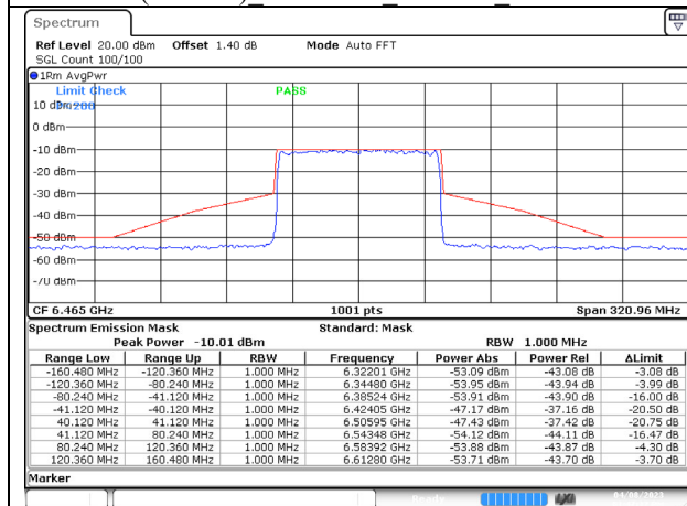
802.11ax (80MHz) 6465MHz Chain A NSS-1
