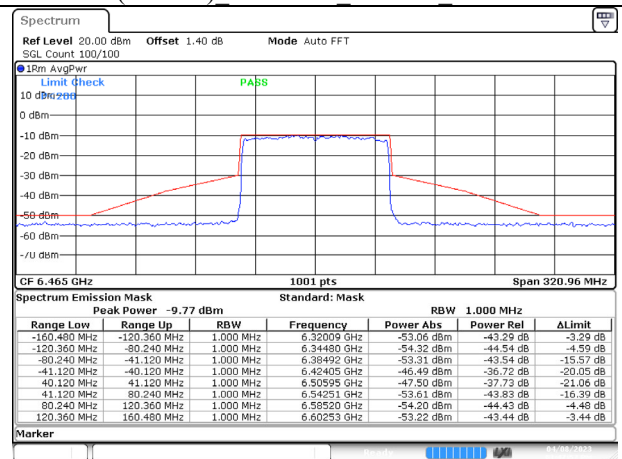
802.11ax (80MHz) 6465MHz Chain B NSS-1
