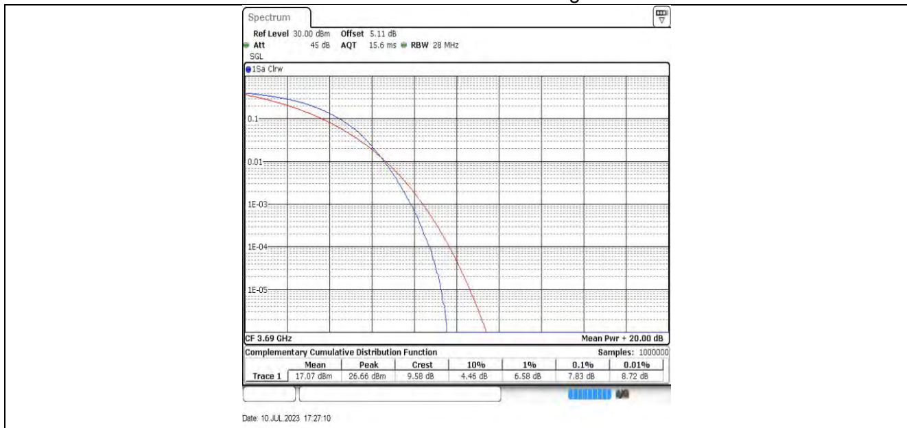
20MHz-56640 64QAM
