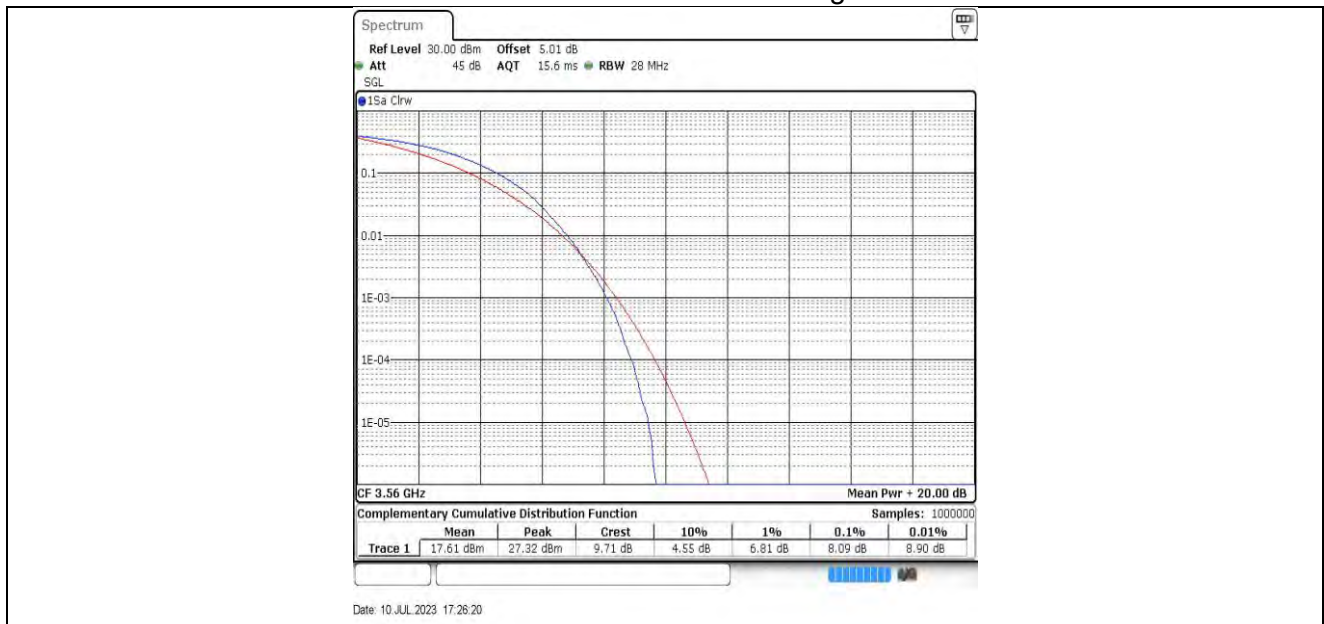
20MHz-55340 64QAM
