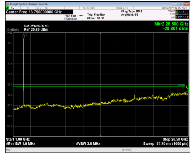
Band7-20MHz-16QAM-20850-1RB#0-Range2:1000~26 500MHz
