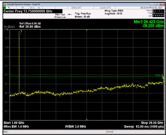
Band41-5MHz-QPSK-41215-1RB#0-Range2:1000~265 00MHz
