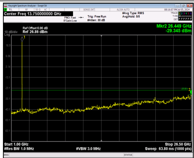
Band7-20MHz-16QAM-21350-1RB#0-Range2:1000~26500MHz
