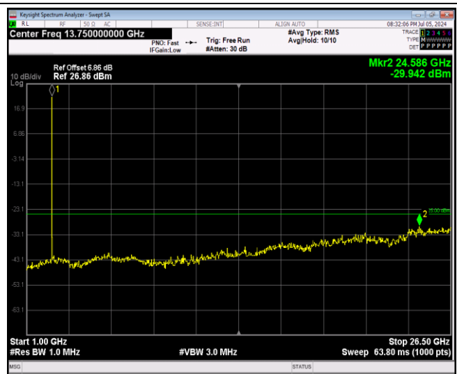
Band41-5MHz-QPSK-40640-1RB#0-Range2:1000~265 00MHz
