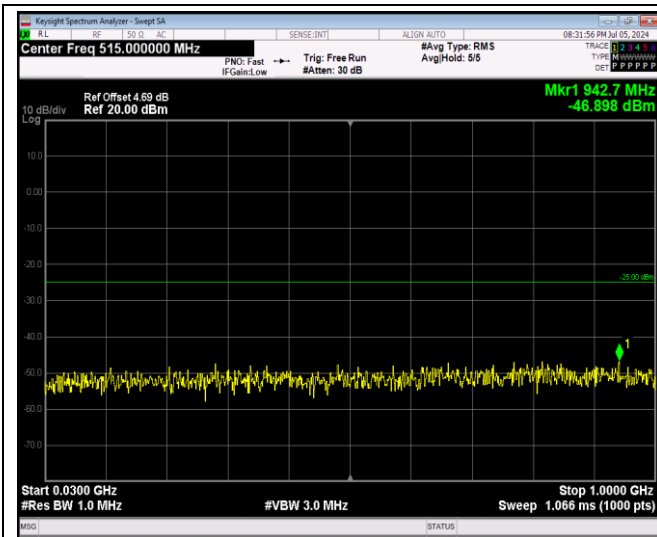
Band41-5MHz-QPSK-40640-1RB#0-Range1:30~100 OMHz
