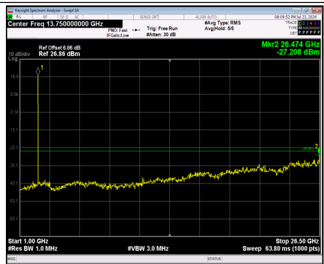
Band7-20MHz-QPSK-20850-1RB#0-Range2:1000~265 00MHz
