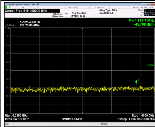
Band41-5MHz-QPSK-41215-1RB#0-Range1:30~100 OMHz
