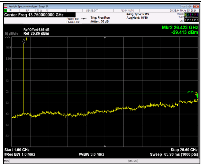
Band41-5MHz-64QAM-40065-1RB#0-Range2:1000~26500MHz
