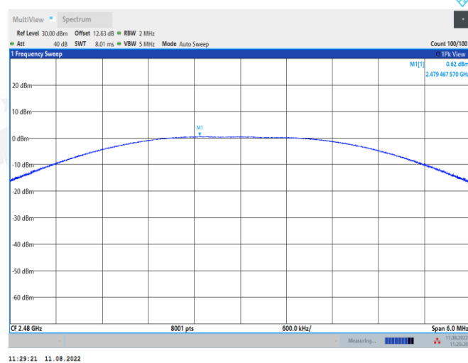
BLE_2M_Ant1_2480
