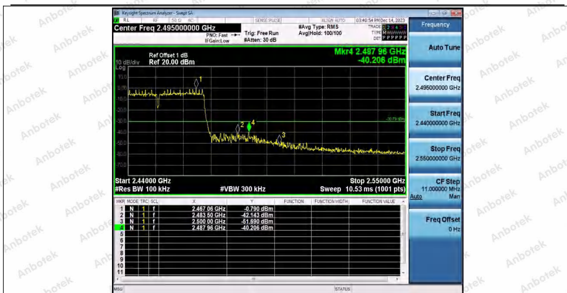
11N40MIMO_Ant2_High_2452
