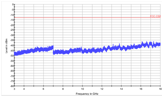
GSM 1900 CH-High 3GHz~18GHz
