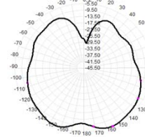
2500.0MHz Total(E2-YZ), Max=-5.58dBi
