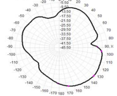
Total(H+V), Max=-7.54dBi, CrD=16.32
