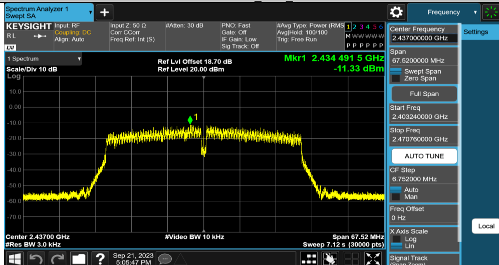
11N40MIMO Ant2 2437
