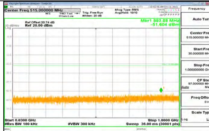
11G_Ant2_2437_30~1000
