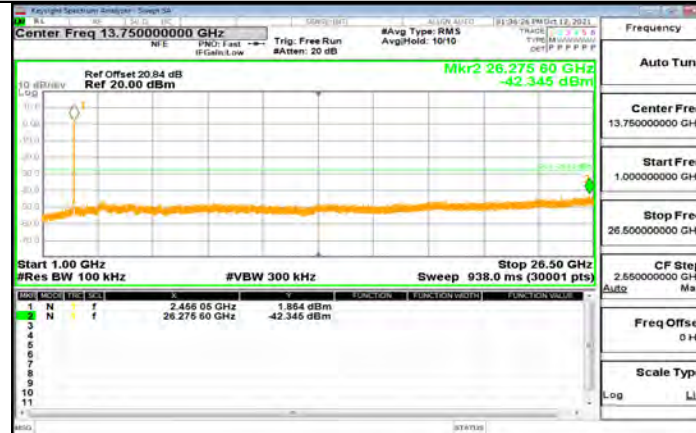
11N40MIMO_Ant1_2452_1000~26500
