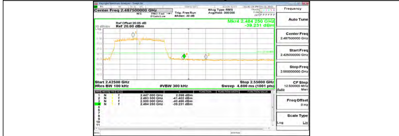
11N40MIMO_Ant2_High_2452
