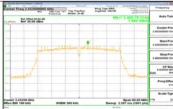
11N40MIMO_Ant1_2452_0~Reference
