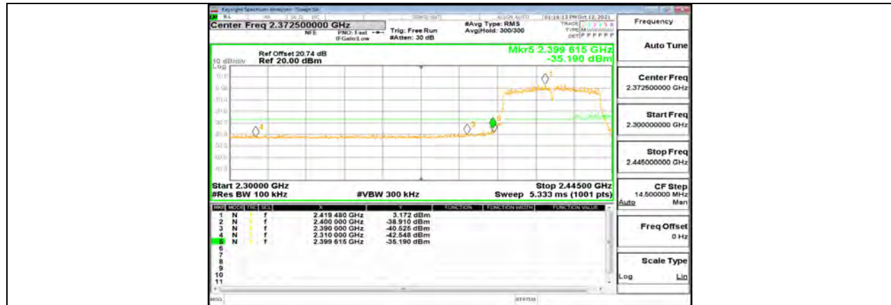
11N40MIMO_Ant2_Low_2422
