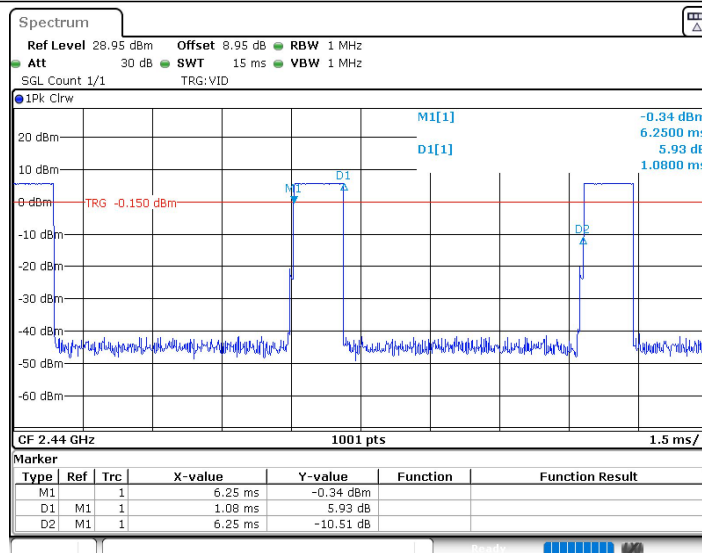
ZIGB_Ant1_2440
