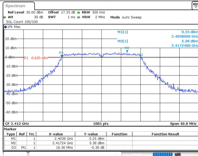
11G_Ant1_2412
