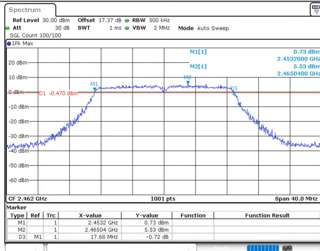
11N20SISO_Ant1_2462
