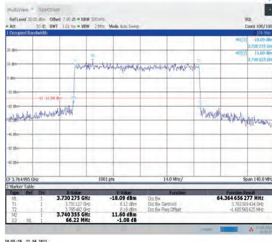
1-N78-3700-3800--30-70-H-3-DFT-16QAM-Outer_Fu ll-180@0-Ant1-64.365-66.220-≤70-PASS
