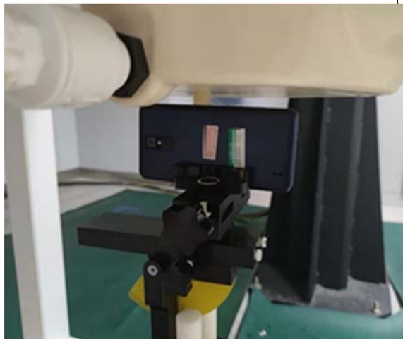
Left(10mm)
