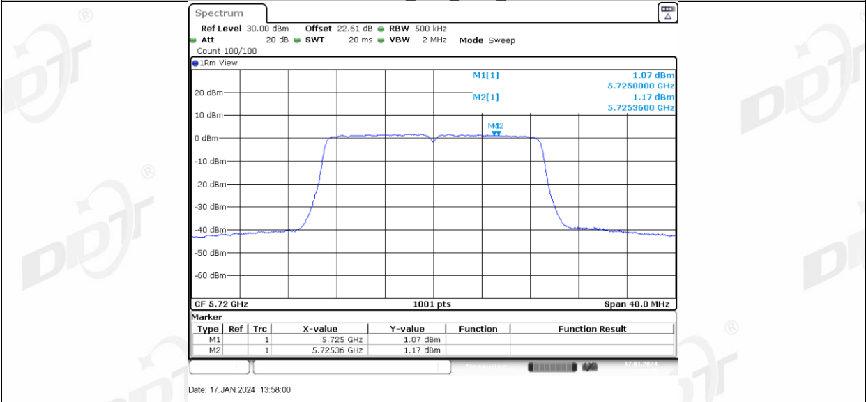
11N20MIMO Ant2 5720 UNII-3
