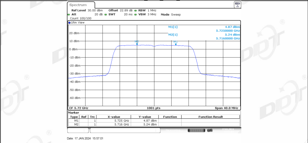
11AC20MIMO Ant1 5720 UNII-3
