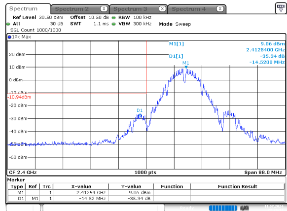
b_2412MHz_Chain 0
