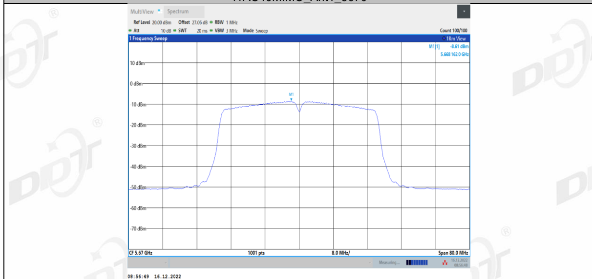
11AC40MIMO_Ant2_5670
