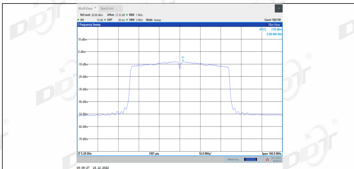
11AC80MIMO_Ant2_5290
