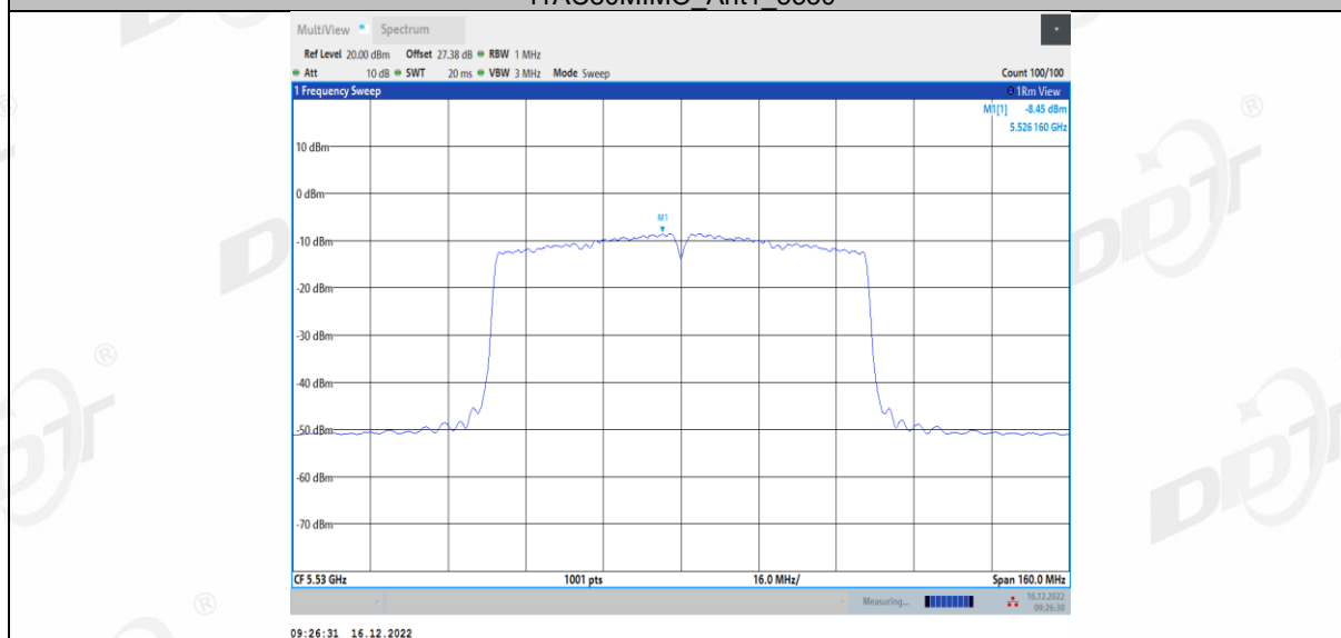
11AC80MIMO_Ant2_5530
