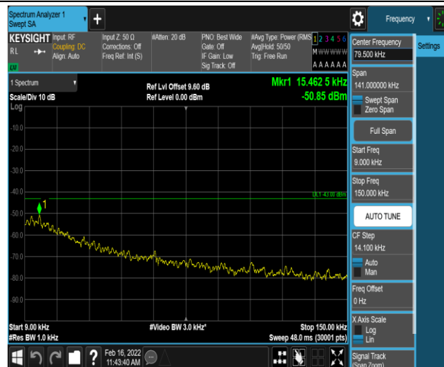
Band66-20MHz-QPSK-132072-1-0-Low-0.009-0.15--50.85-PASS
