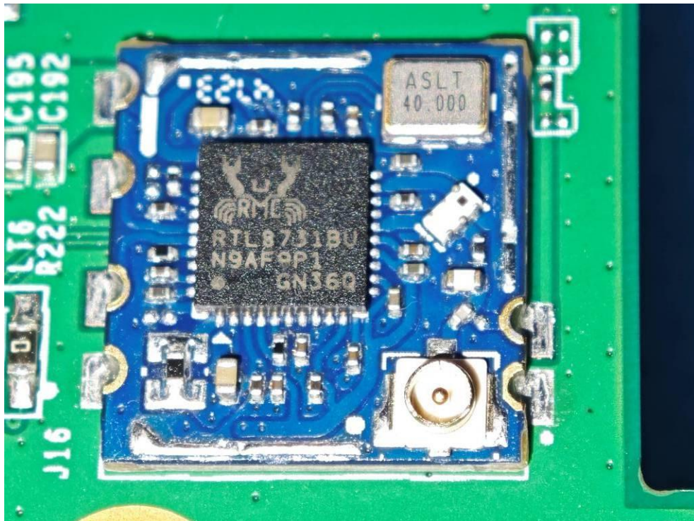
Wi-Fi module 2
