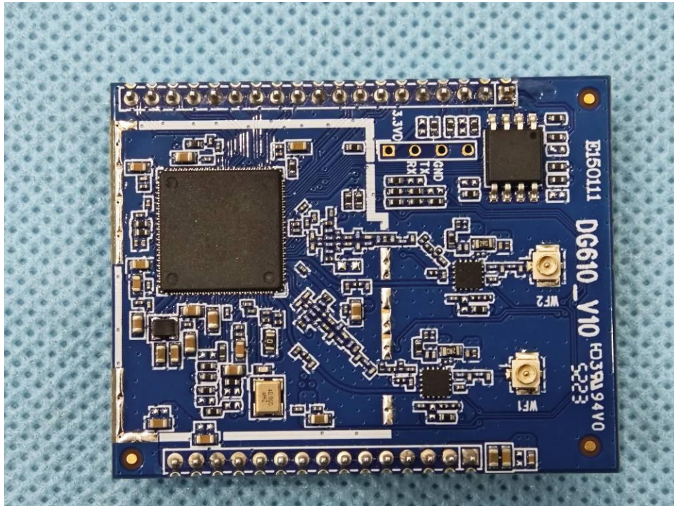
Wi-Fi module 1
