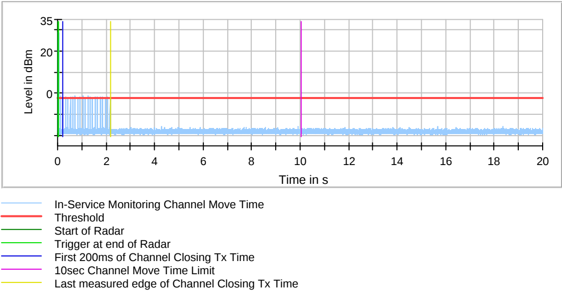
802.11ac VHT80 5530MHz
