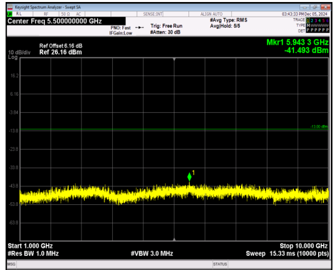
Band26-1.4MHz-QPSK-26797-1RB#0-Range2:1000~10000MHz
