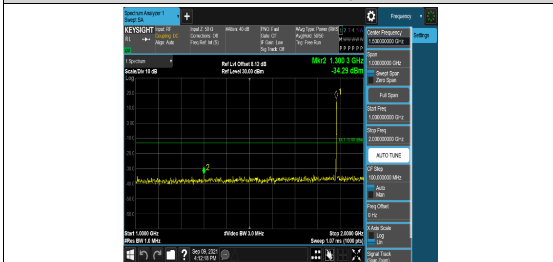
Band25-3MHz-QPSK-26365-1RB#0-Range4:1000~2000MHz
