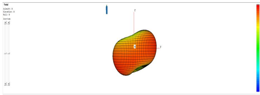
GSM 850
