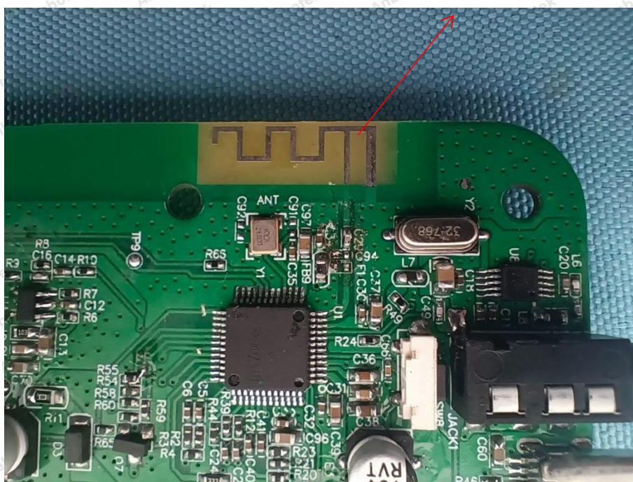
RX ANT
