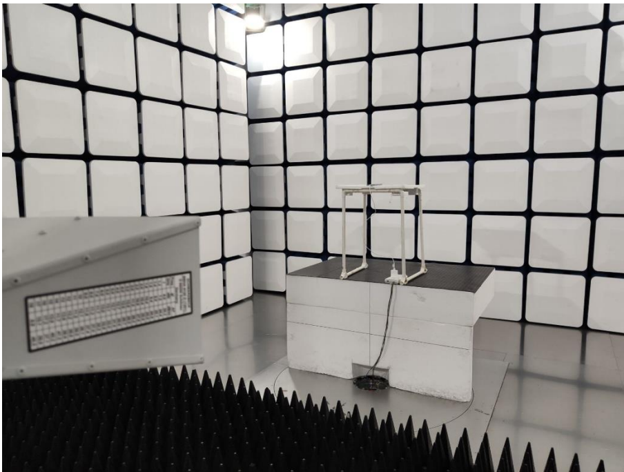
Above 1GHz-BT/WIFI
