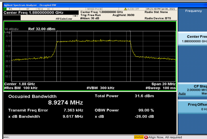
Band2-10MHz-QPSK-18900-50RB#0-8.9274
