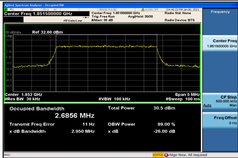
Band2-3MHz-16QAM-18615-15RB#0-2.6856
