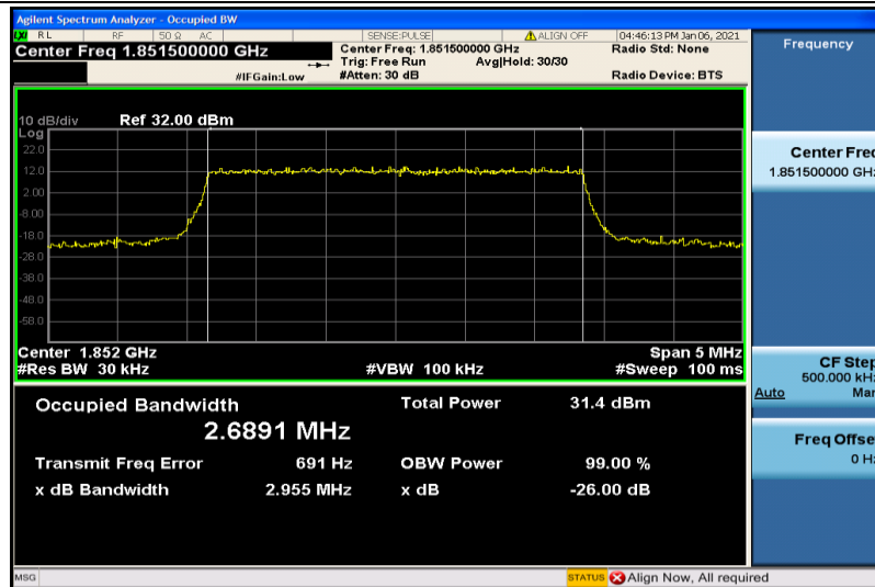
Band2-3MHz-QPSK-18615-15RB#0-2.6891
