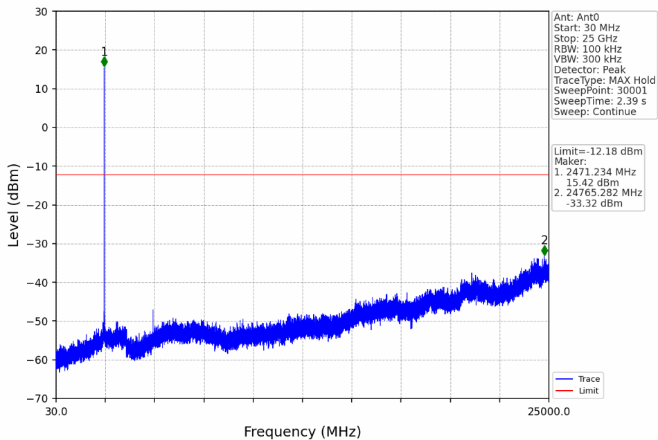
1.4M_HCH_2471.12MHz_Ant0_NTNV
