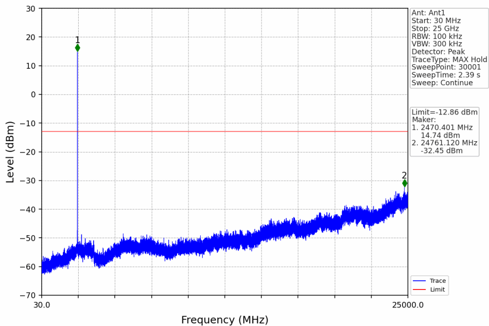
1.4M_HCH_2471.12MHz_Ant1_NTNV
