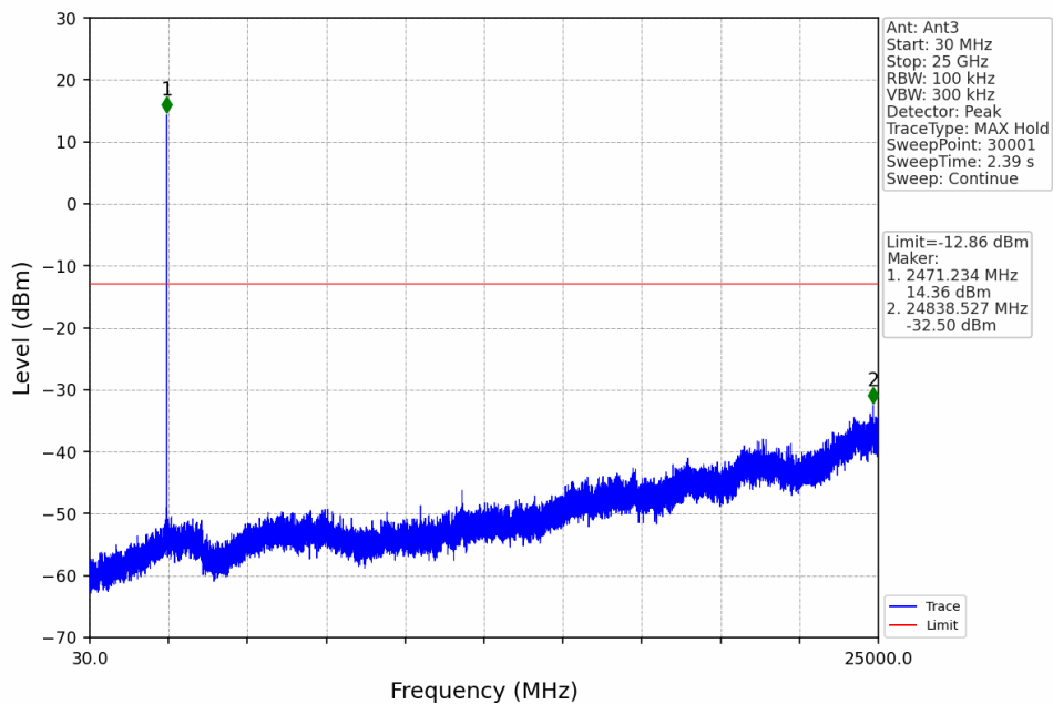
1.4M_HCH_2471.12MHz_Ant3_NTNV
