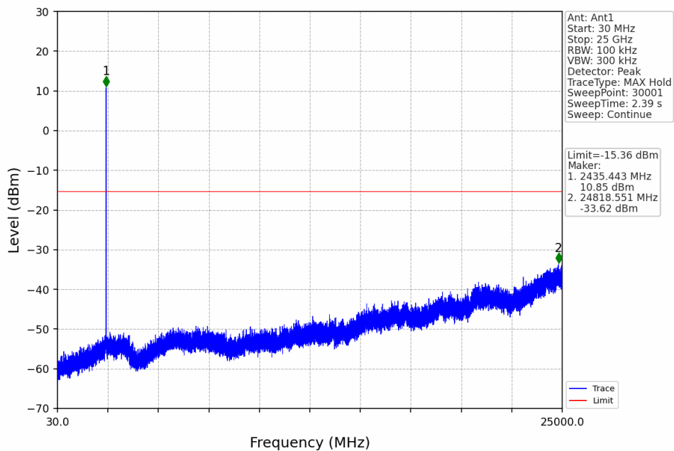
3M_MCH_2435.5MHz_Ant1_NTNV
