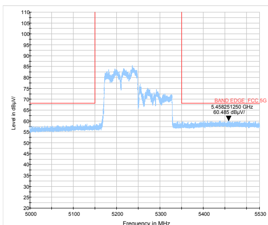
802.11ac VHT80+80 –Channel 42+58: Peak
