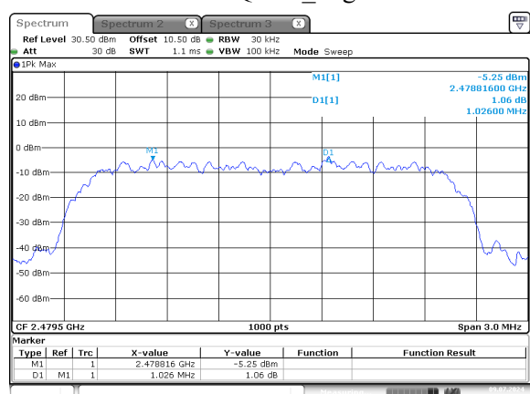
\pi/4 -DQPSK_High
