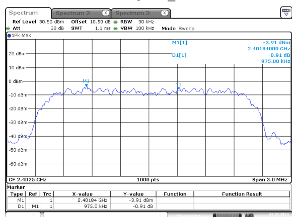
\pi/4 -DQPSK_Low
