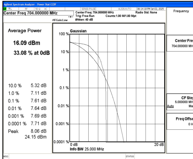
Band12-10MHz-QPSK-23060-1-0-Low-7.61-&lt;=13-PASS
