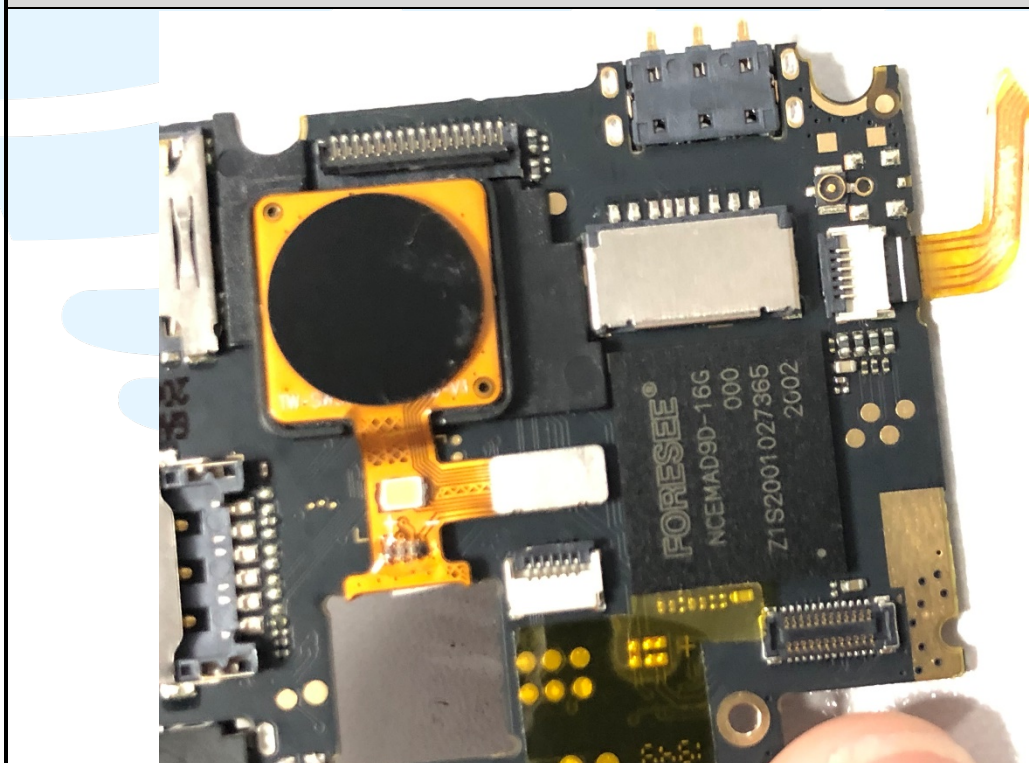
EUT Photo
