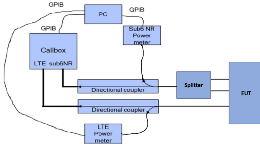
(d) Appendix A – Test Setup Photo 10
